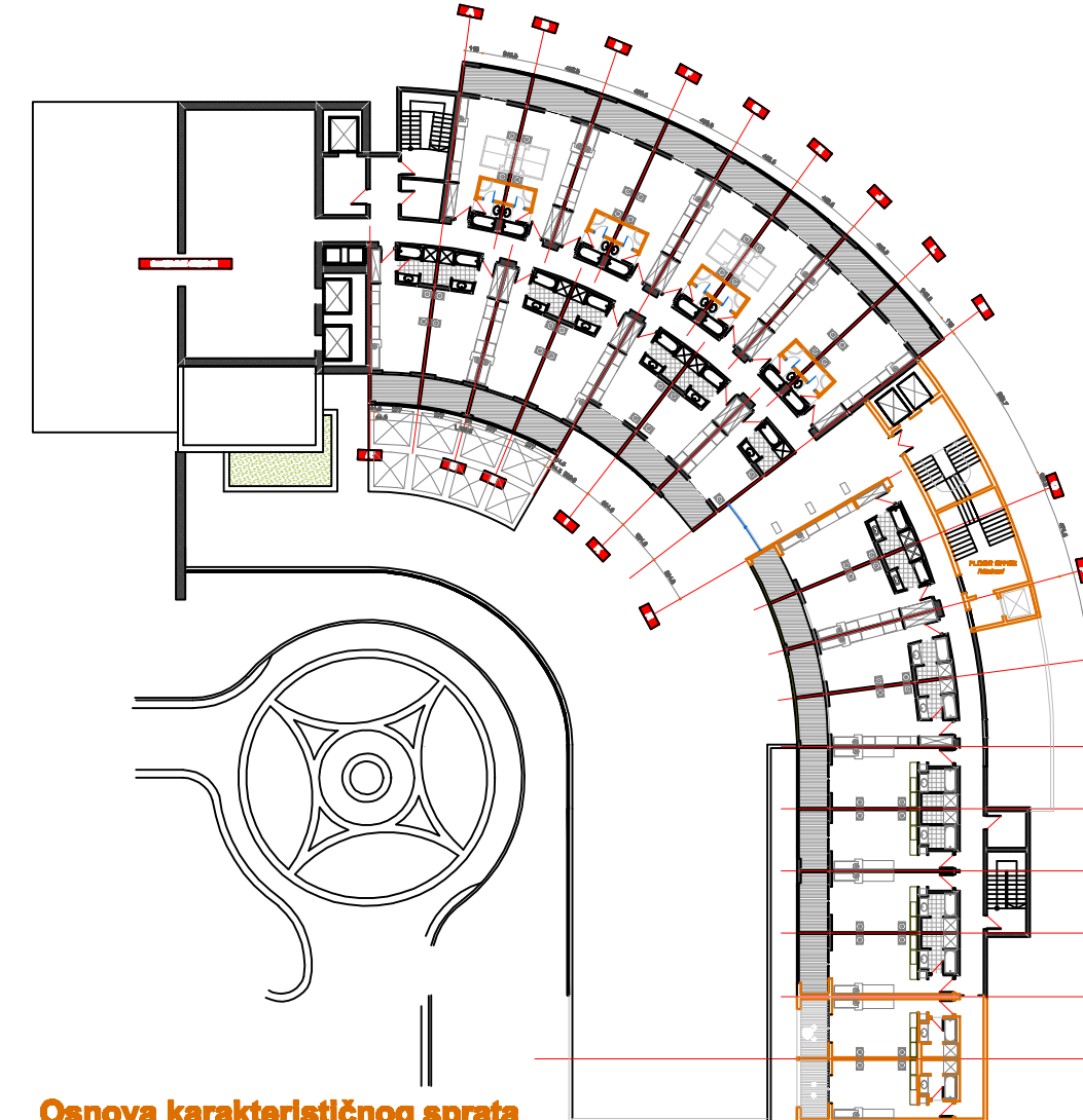
Osnova karakterističnog sprata
