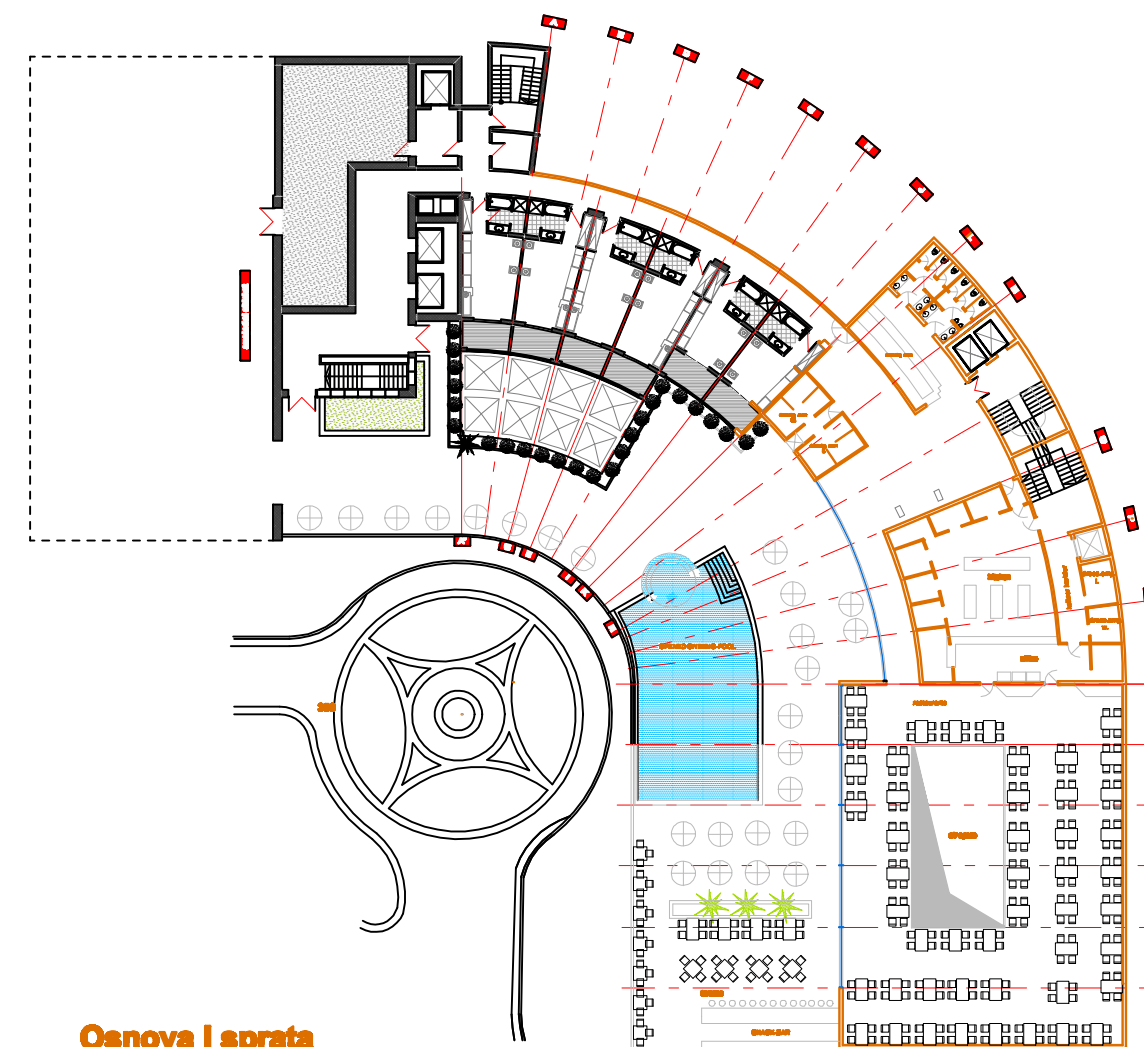
Osnova I sprata
