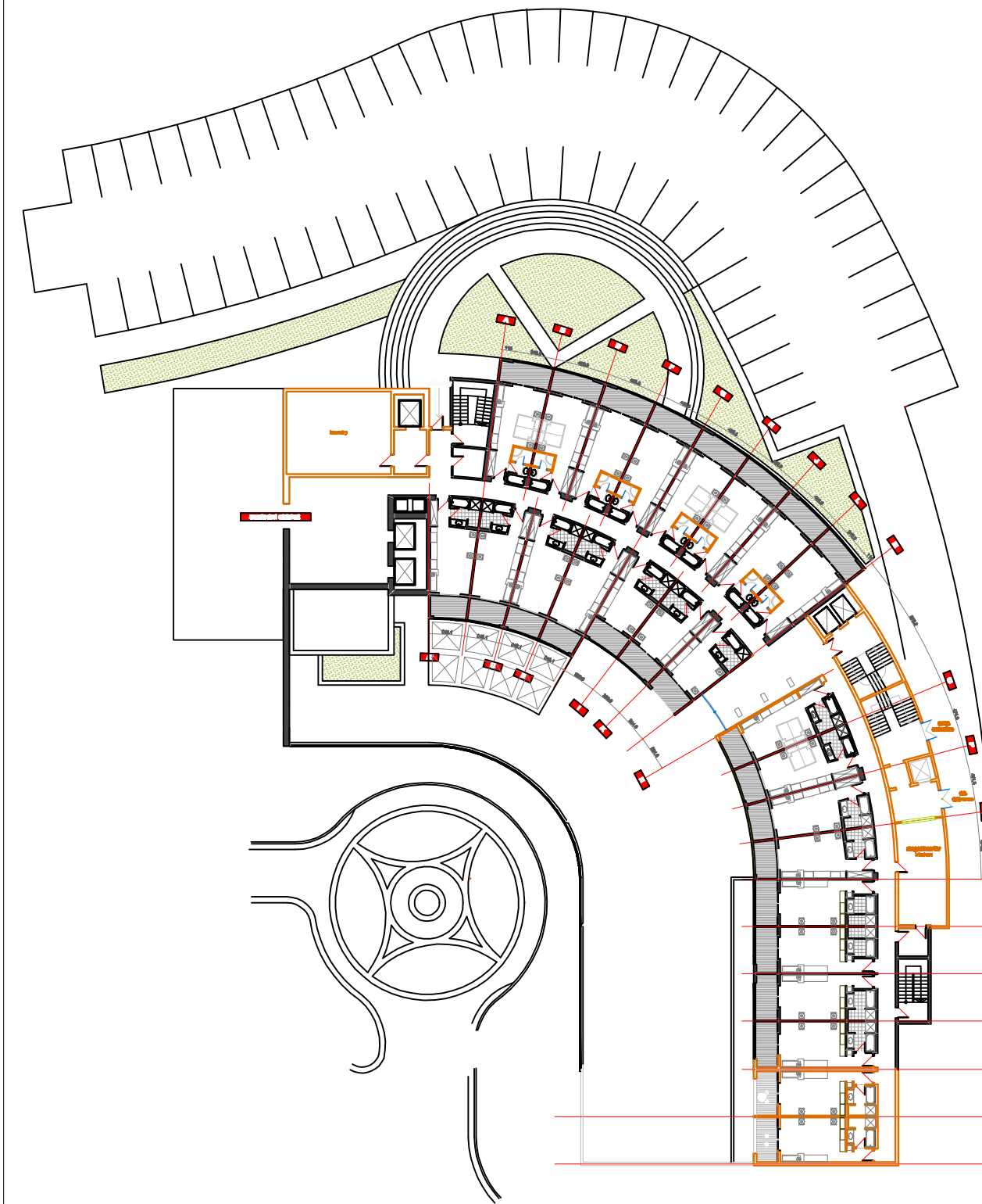
Osnova II sprata
